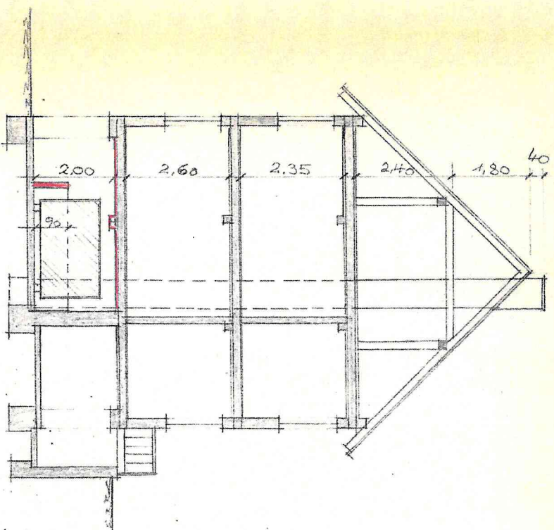
Querschnitt A-B
